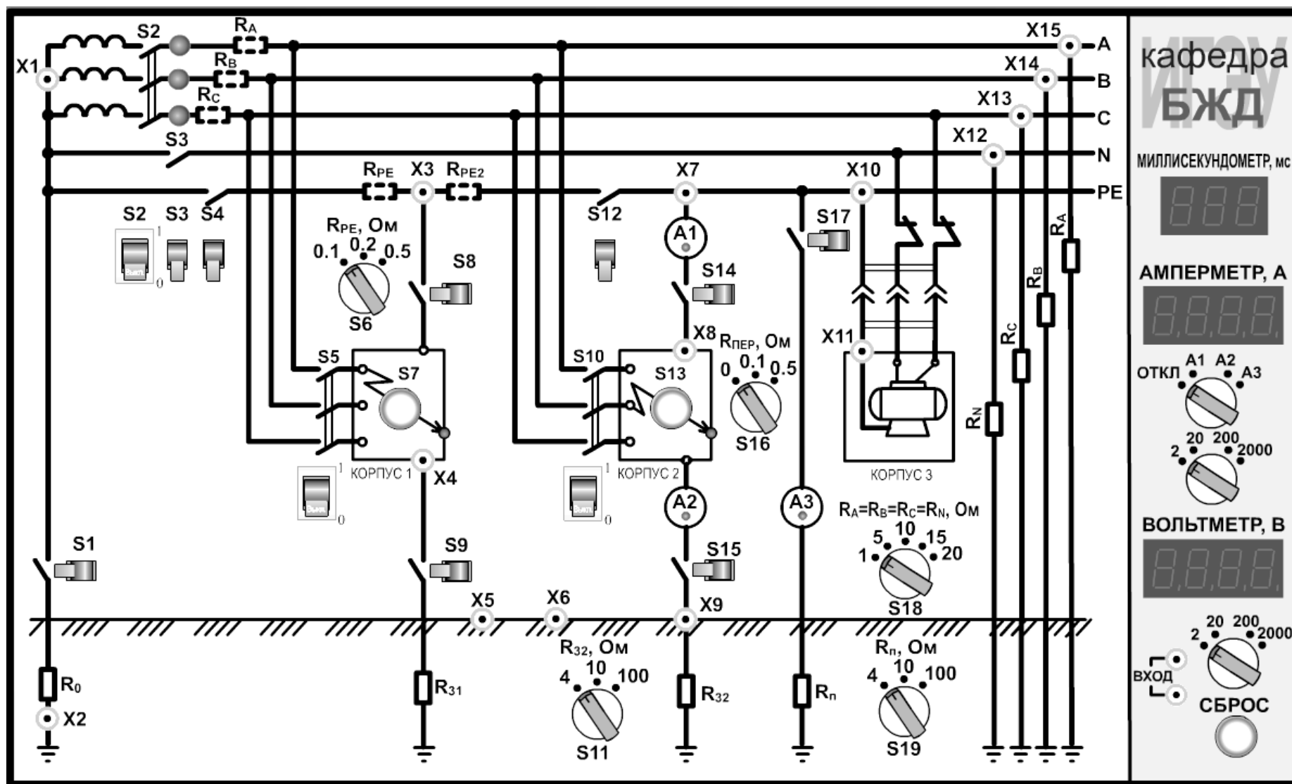
Рис. 8.1. Лицевая панель стенда БЖ 6/2
