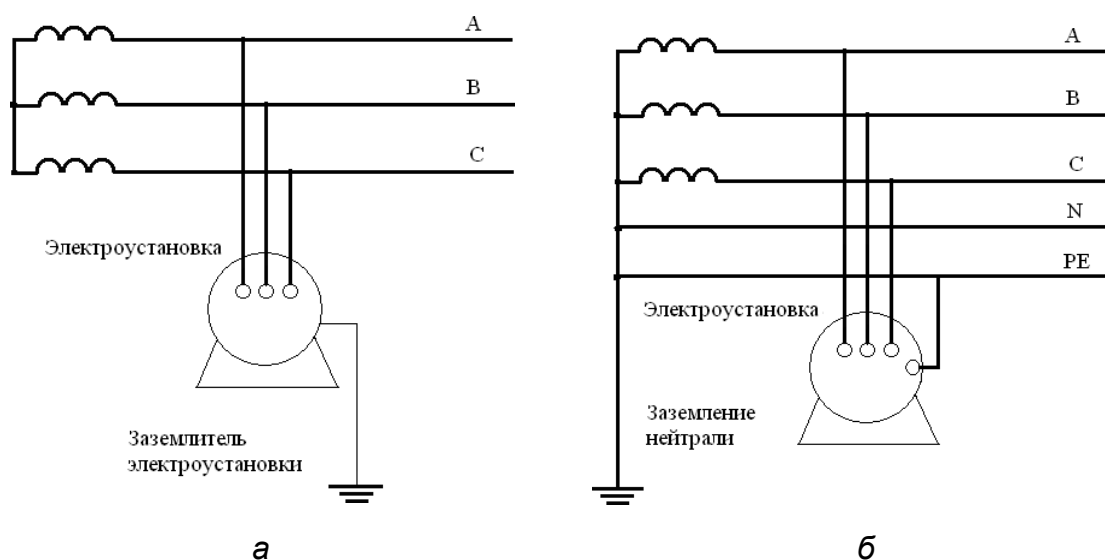
Рис. 8.2. Схемы трёхфазных сетей:
