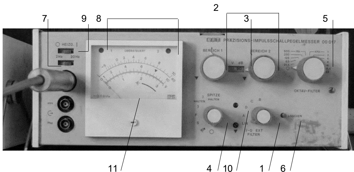
Рис. 6.1. Лицевая панель шумомера _____
