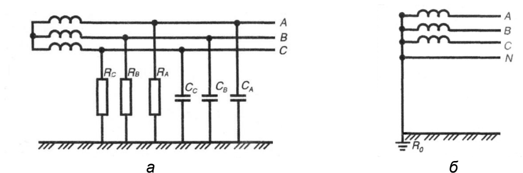
Рис. 7.2. Схемы трёхфазных сетей:
