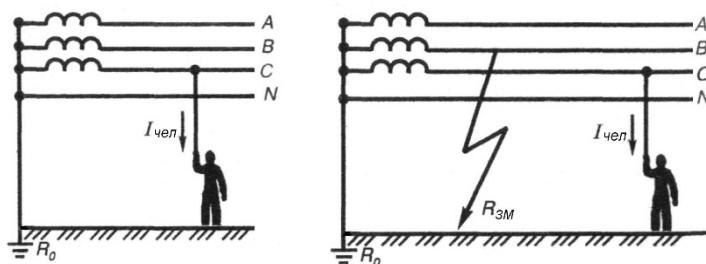
Рис. 7.4. Схемы однофазного включения человека в трёхфазную ____-проводную сеть с _____
