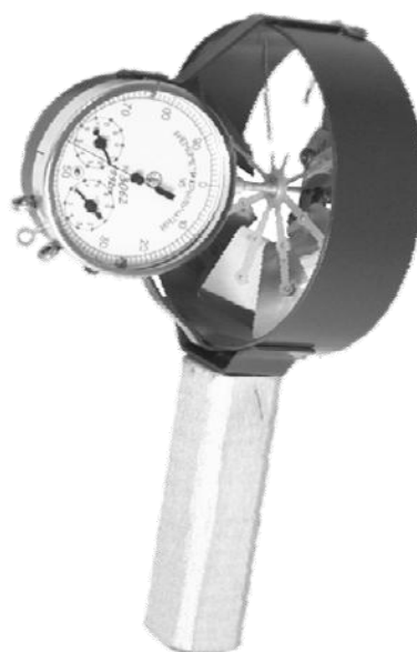
Рис. 2.4. Анемометр крыльчатый
